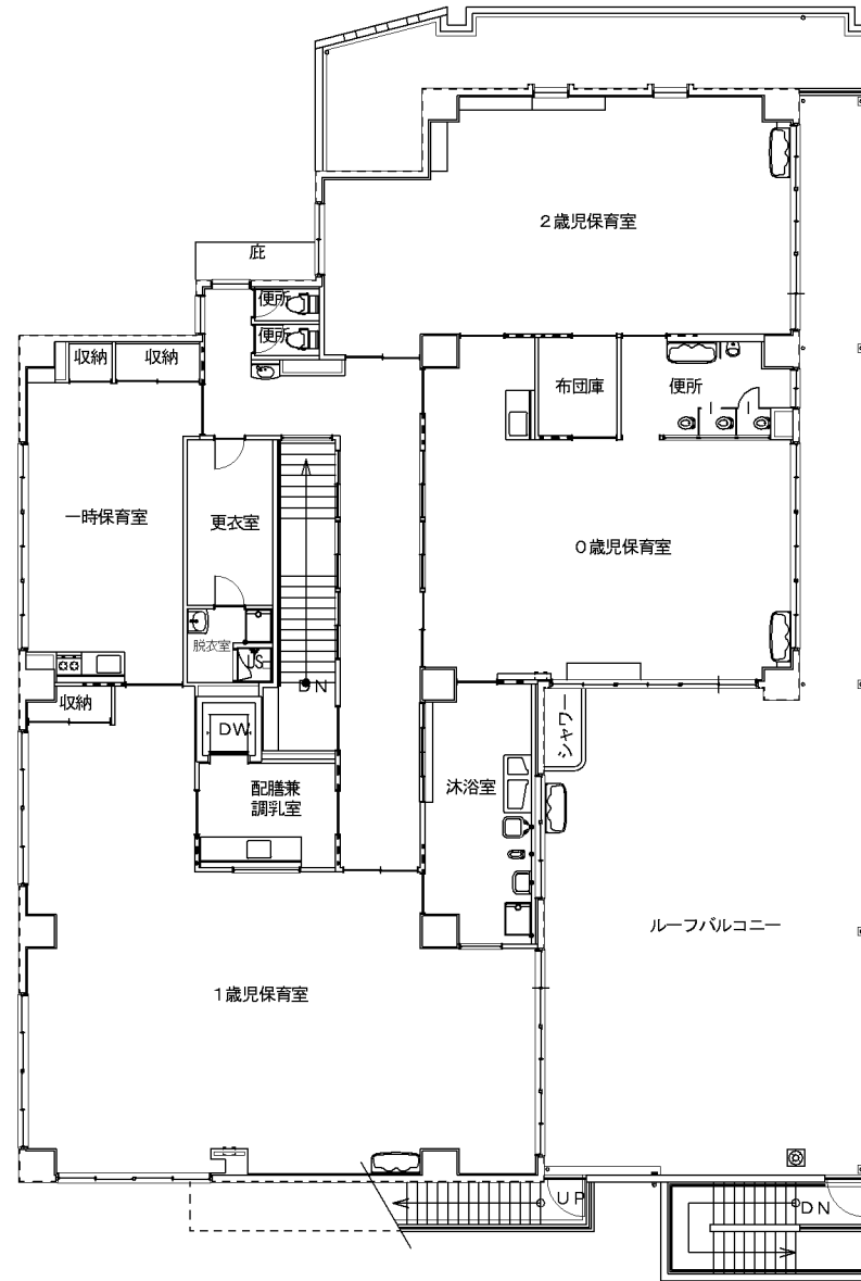
2階 平面図
