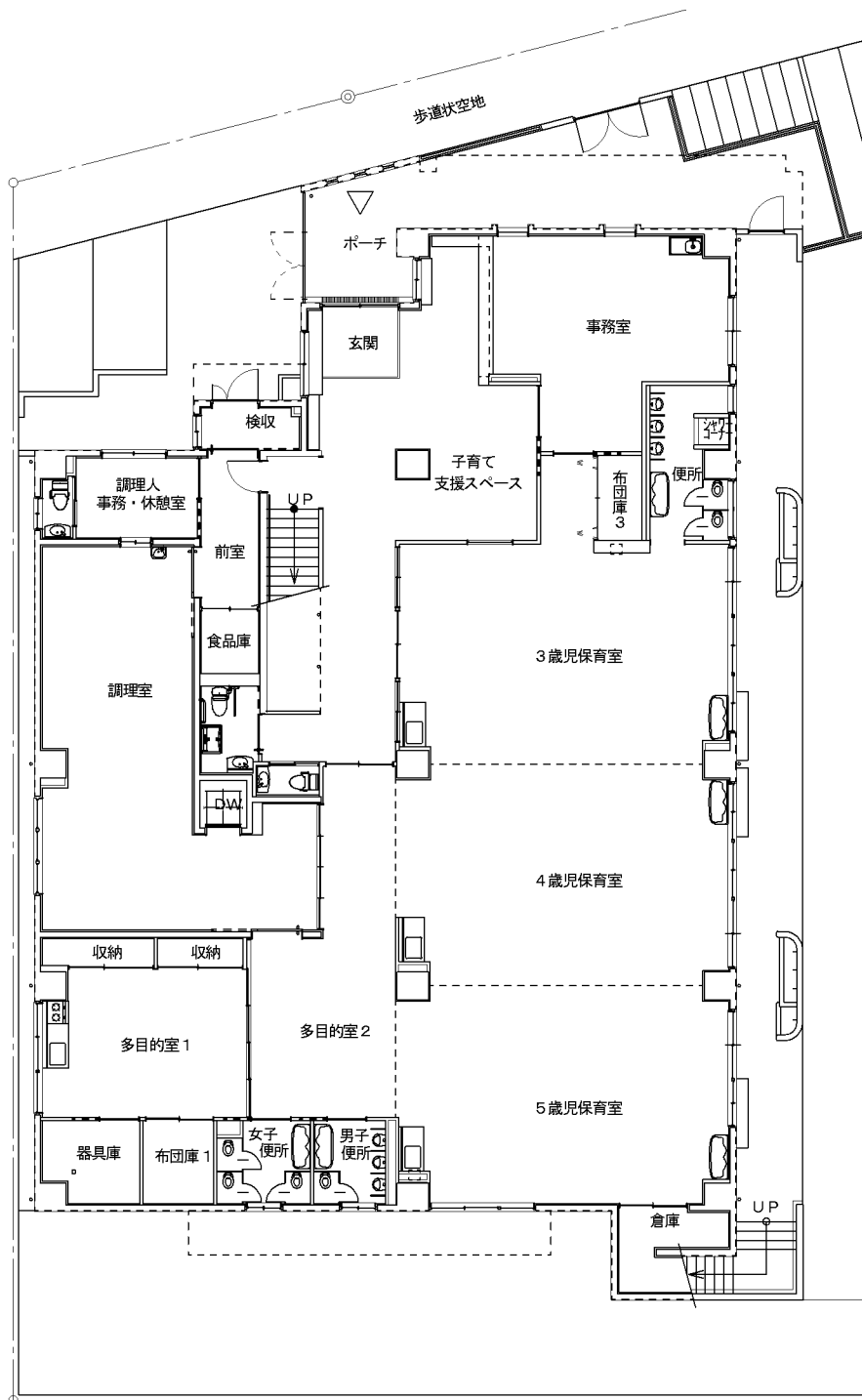
1階 平面図
